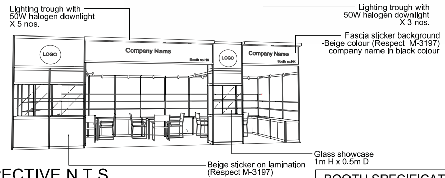
PERSPECTIVE N.T.S
