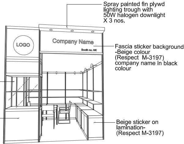
PERSPECTIVE N.T.S.
