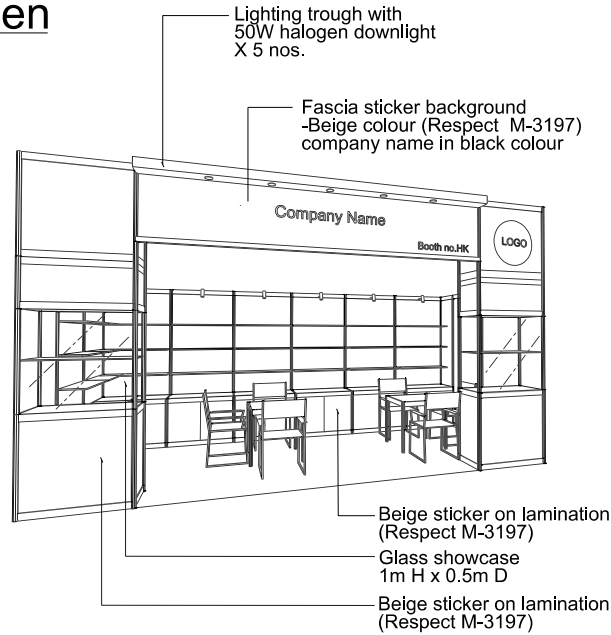
PERSPECTIVE N.T.S
