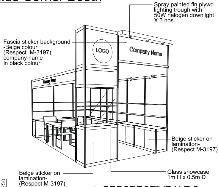
PERSPECTIVE N.T.S
