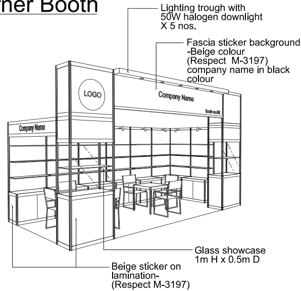
PERSPECTIVE N.T.S.
