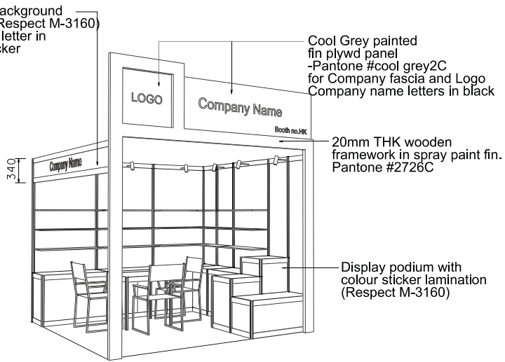
PERSPECTIVE N.T.S
