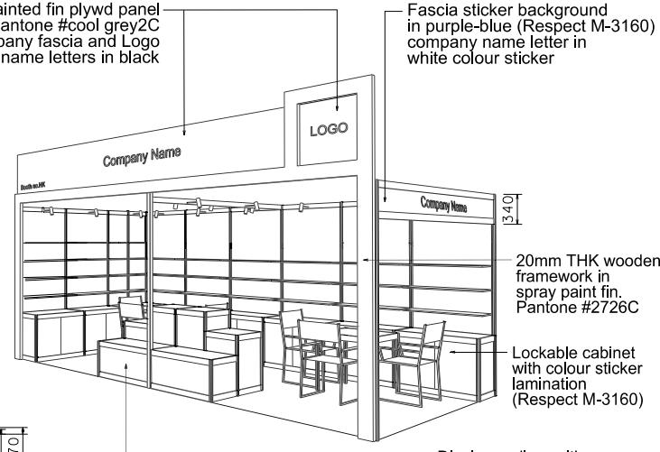
PERSPECTIVE N.T.S
