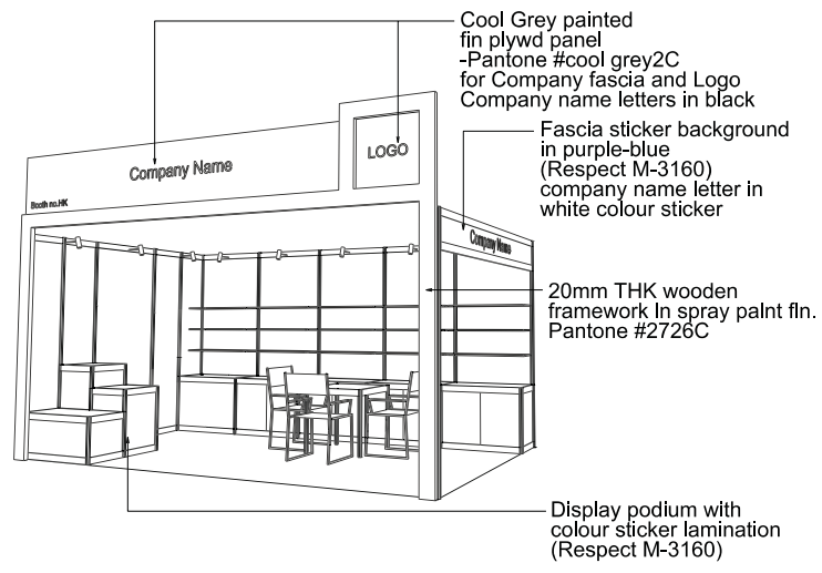
PERSPECTIVE N.T.S
