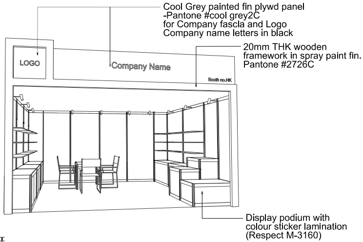
PERSPECTIVE N.T.S
