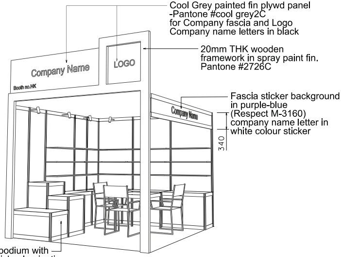
PERSPECTIVE N.T.S
