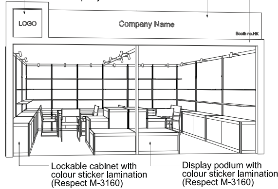
PERSPECTIVE N.T.S
