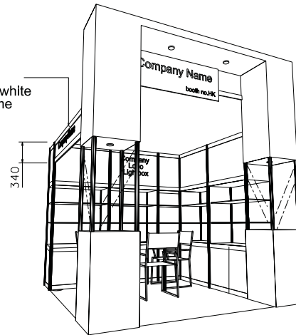
PERSPECTIVE N.T.S
