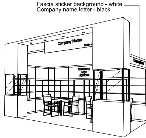
PERSPECTIVE N.T.S.
