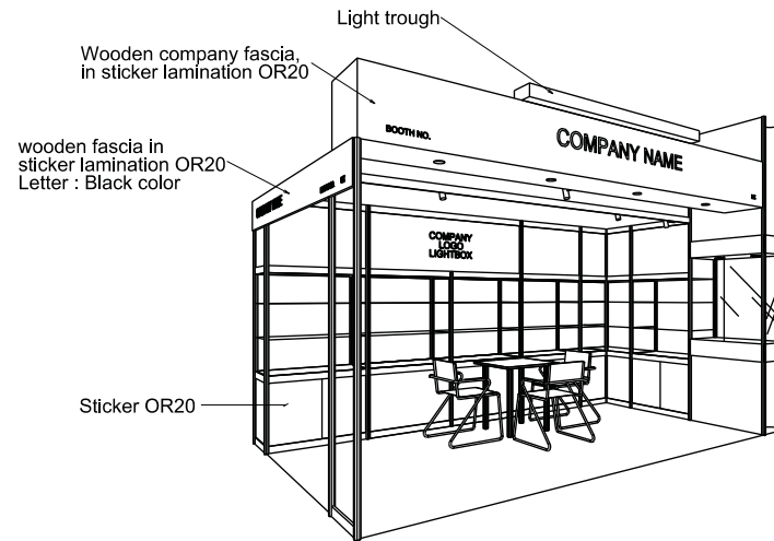
PERSPECTIVE N.T.S
