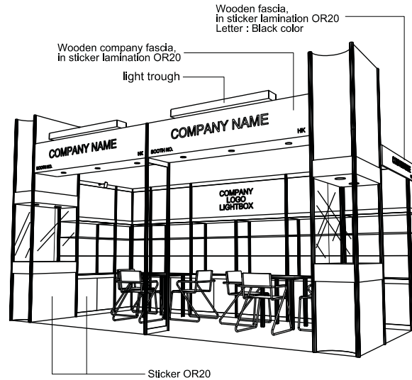
PERSPECTIVE N.T.S.
