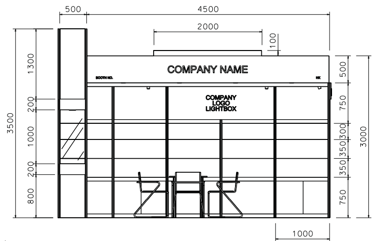
Top Elevation
