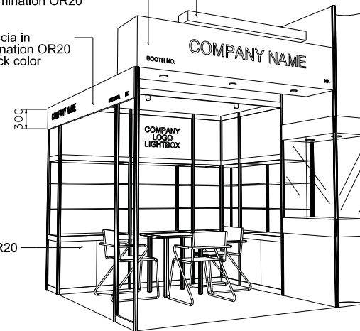
PERSPECTIVE N.T.S
