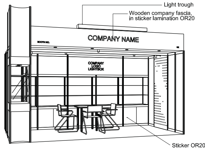
PERSPECTIVE N.T.S
