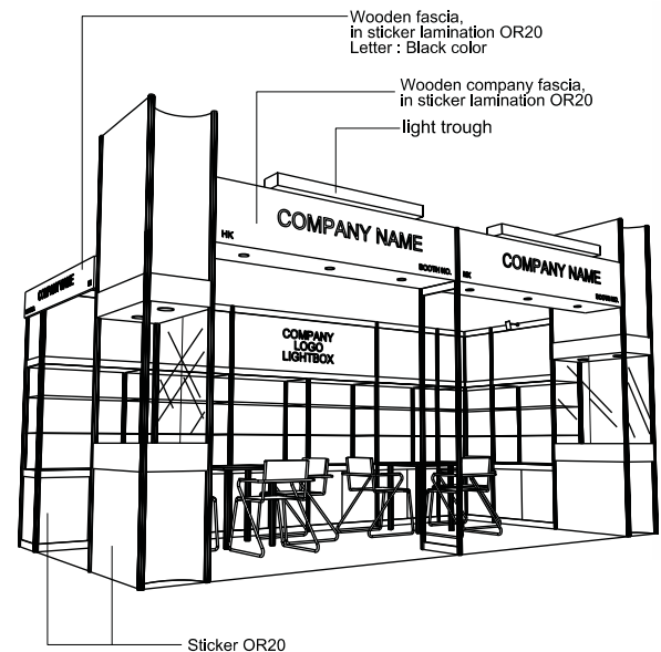
PERSPECTIVE N.T.S.
