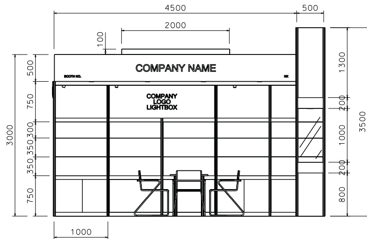
Top Elevation
