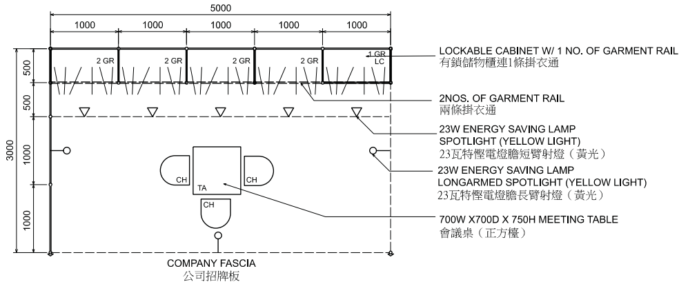
PLAN 平面圖
