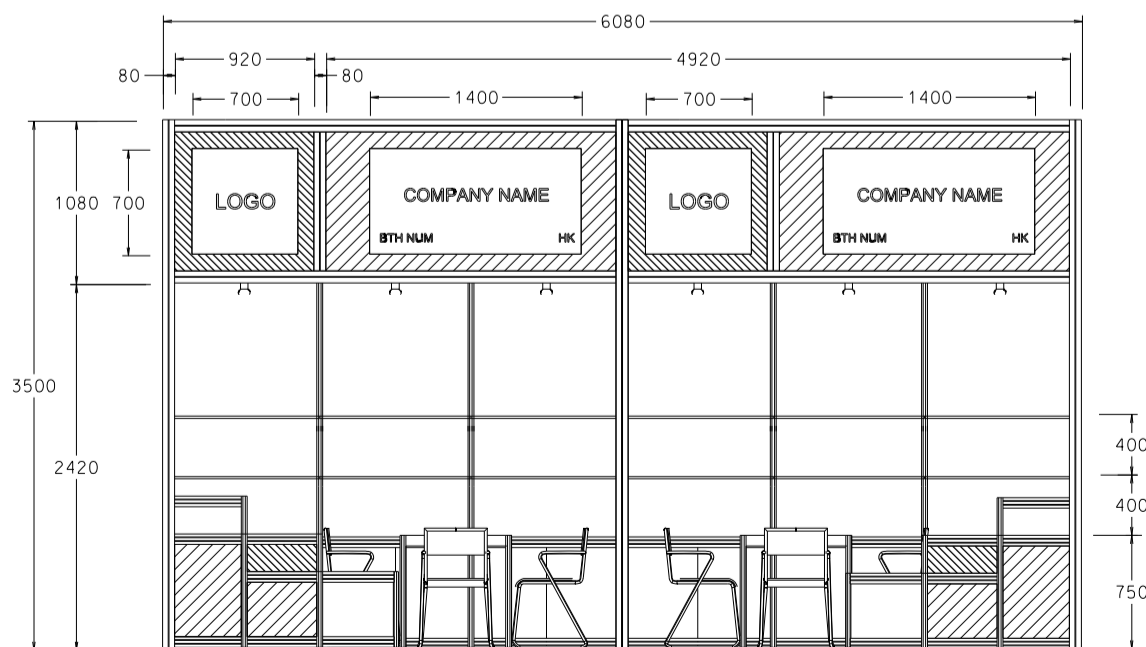
ELEVATION
